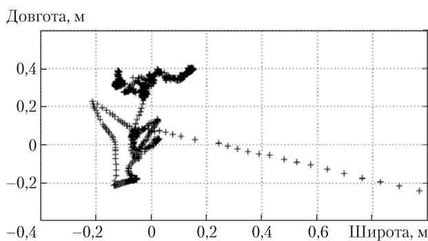
Рис. 11. Нев'язки DGPS-рішення по планових координатах. Розрахункові планові координати. Відстань 20 км
