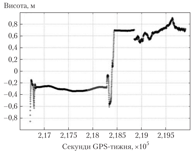
Рис. 16. Нев'язки DGPS-рішення по висоті. Розрахункова висота. Відстань 60 км
