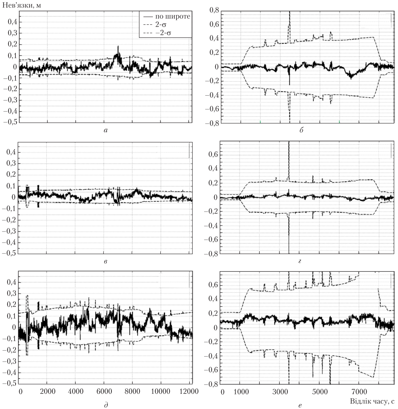
Рис. 5. Нев'язки отриманого WL-рішення відносно еталонних оцінок та апіорна оцінка точності рішення, розрахована за моделлю похибок, для спостережень на борту гелікоптера ( a , в , д ) і на борту літака ( б , г , е )
