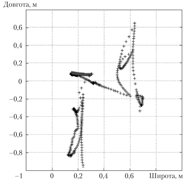
Рис. 15. Нев'язки DGPS-рішення по планових координатах. Розрахункові планові координати. Відстань 60 км
