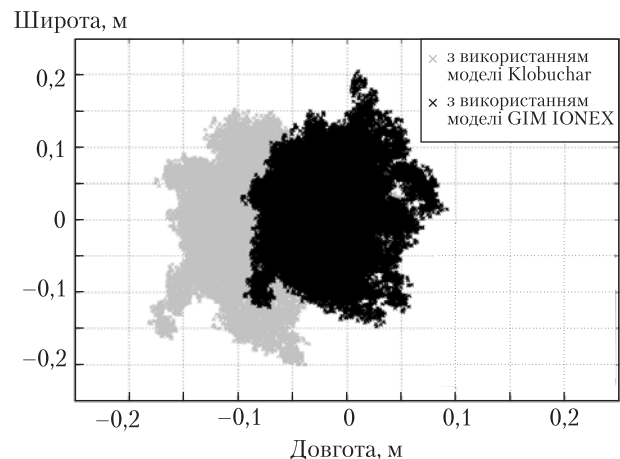
Рис. 4. Відхилення оцінок планових координат станцій PRYL від еталонних значень при обробці спостережень відносно станції GLSV
