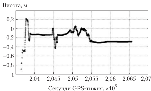
Рис. 12. Нев'язки DGPS-рішення по висоті. Розрахункова висота. Відстань 20 км
