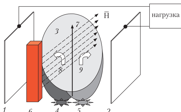
Рис. 2. Иллюстрация работы и назначения элементов предлагаемой ячейки магнитного типа: 1 – анод; 2 – катод; 3 – область реакции; 4 – устройство подачи топлива; 5 – устройство подачи окислителя; 6 – источник магнитного поля. Стрелка 7 указывает исходное направление движения топлива, окислителя и продуктов реакции, стрелки 8 и 9 – направление отклонения зарядов
